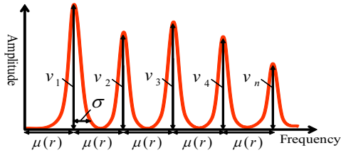
図2 周波数エンベロップ
