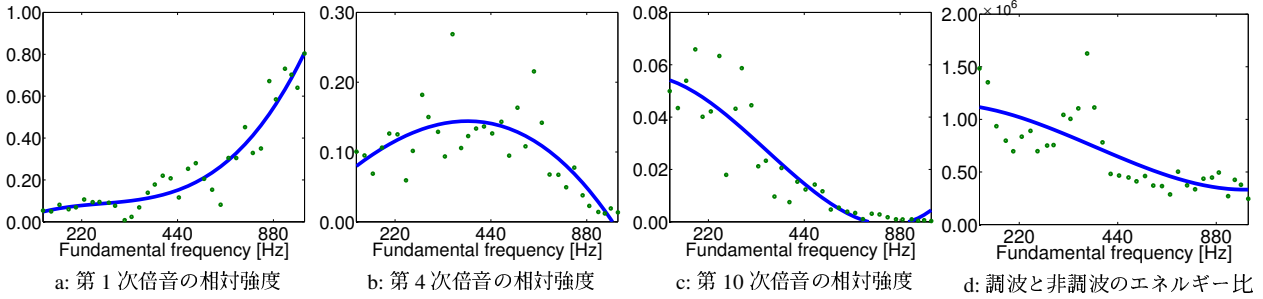
図4 トランペットの音高依存特徴関数. 点と実線はそれぞれ、音高ごとに分析された音色の特徴量と、導出された音高依存特徴関数である。
