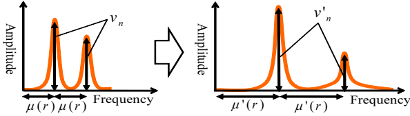
図6 周波数エンベロープの操作
