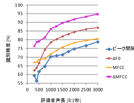
図 5 アクセントピーク間隔， \Delta F0 ，MFCC， \Delta MFCC を利用した場合の識別精度と音声長の関係
