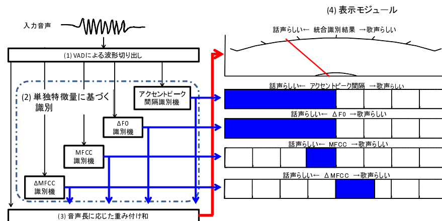
図9 左：デモアプリケーション概要図。右：表示例。一番上が最終的な識別尤度差（連続値）を示し、下の4つが特徴量毎の識別結果（尤度差）を示す。中央より左にいくほど話声尤度のほうが高いことを示し、右にいくほど歌声尤度のほうが高いことを示す。この表示例は話声を入力したもので、 \Delta MFCC が歌声だと誤識別（歌声のほうが尤度が高い）しているが、他の特徴量では話声の尤度が高いため、統合結果も話声の尤度が高くなることを示している。
