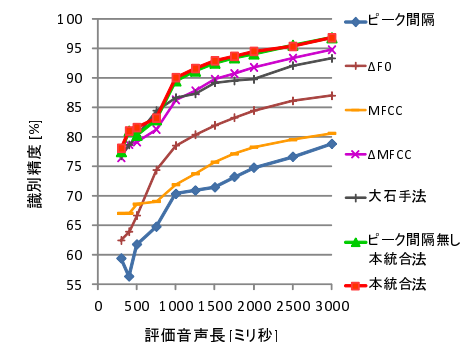
図 6 全ての手法の識別精度と音声長の関係
