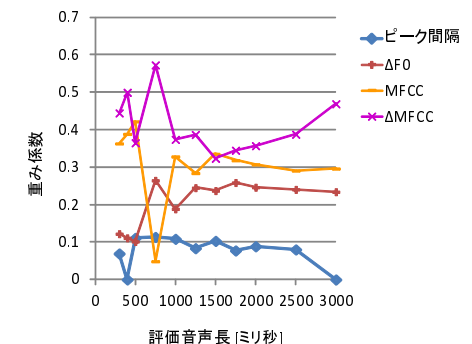
図 8 本統合法に用いた重み係数と入力音声長の関係
