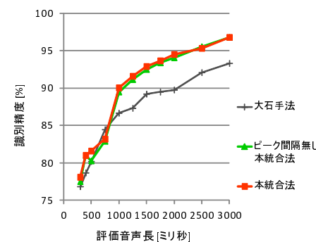
図 7 従来手法・本手法による統合方法と音声長の関係
