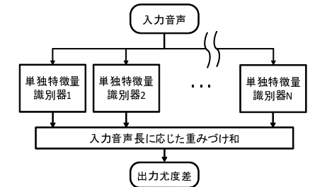
図 4 本統合手法．各単独特徴量識別器の出力を入力音声長に応じた重み付けた和をとる．
