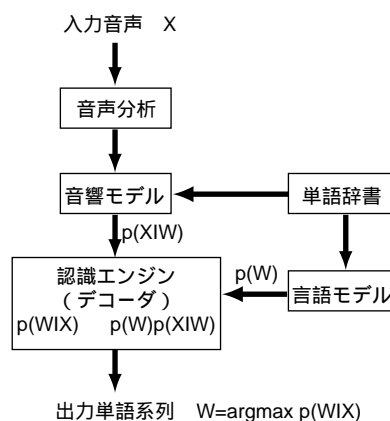
図-1 音声認識システムの構成
