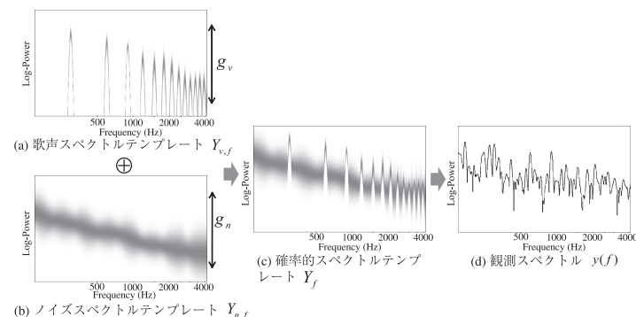
図 1 観測スペクトルの生成過程. 図の濃淡は確率密度を表現する. 重みパラメータ g_v と g_n を調整することで, 様々な SIR のスペクトルを表現できる
