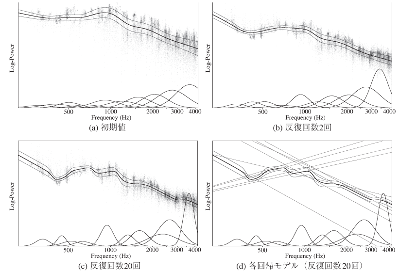
図5 混合回帰モデルのパラメータ推定の過程の一例。 t は反復回数を表す。各図の中心の太い線は混合回帰モデルの平均を表し、その上下の細い2本の線は標準偏差を表す。背景の細かい点は学習データの調波成分を表し、各図の下部の複数の山は、ゲート関数を構成する各ガウス分布とその重みの積 \psi_m \mathcal{N}(f; \mu_m, \sigma_m^2) を表す
