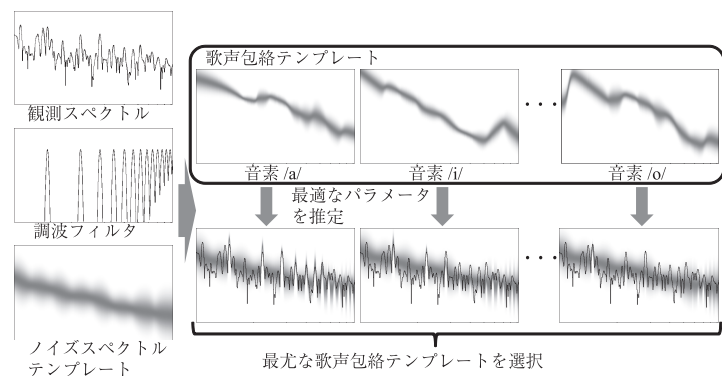
図 4 音素認識方法の概要
