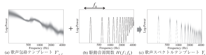
図 2 歌声スペクトルテンプレートの例. 歌声包絡テンプレートと駆動音源関数から生成される
