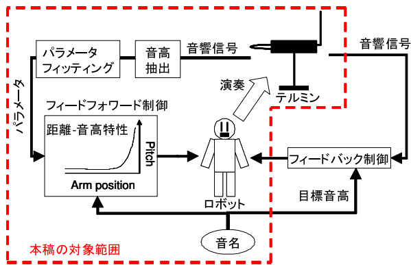
図 1: システム図: 破線で囲んだ範囲が本稿の対象
