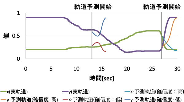
図 5: 確信度と物体軌道の時間変化
